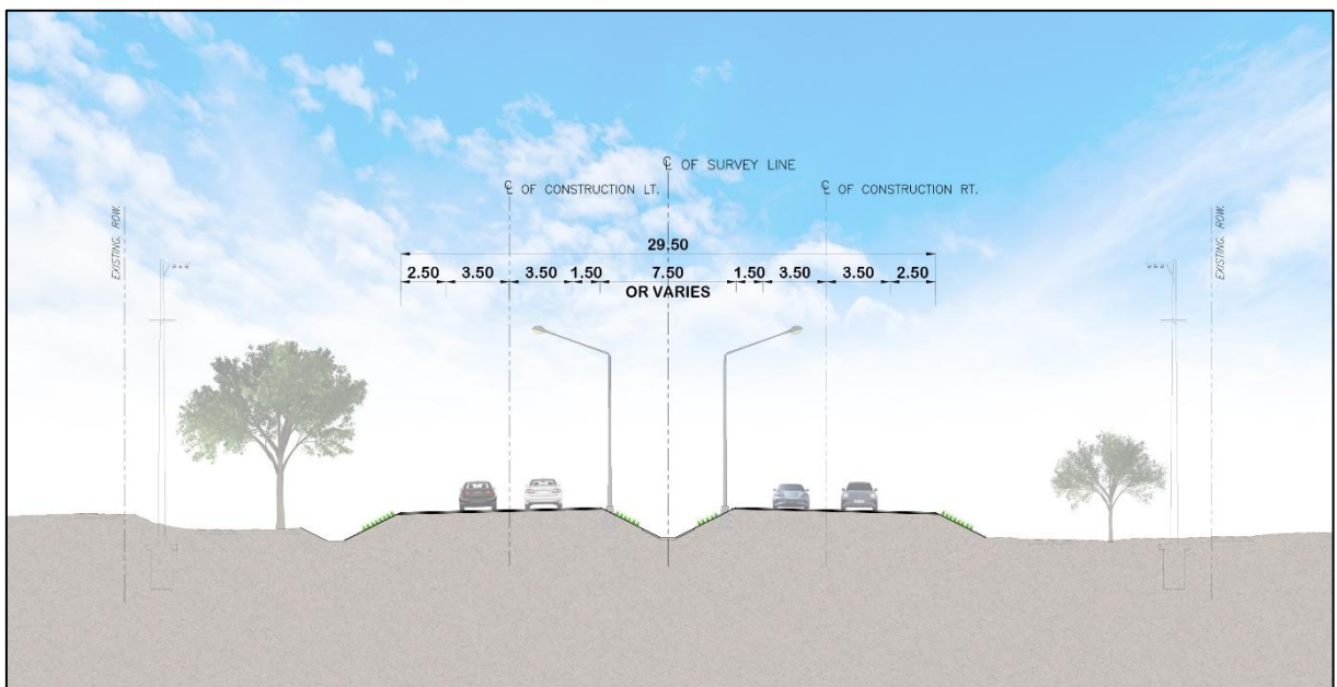
รูปที่ 5.1-1 รูปแบบปรับปรุงทางหลวง 4 ช่องจราจรเดิม
