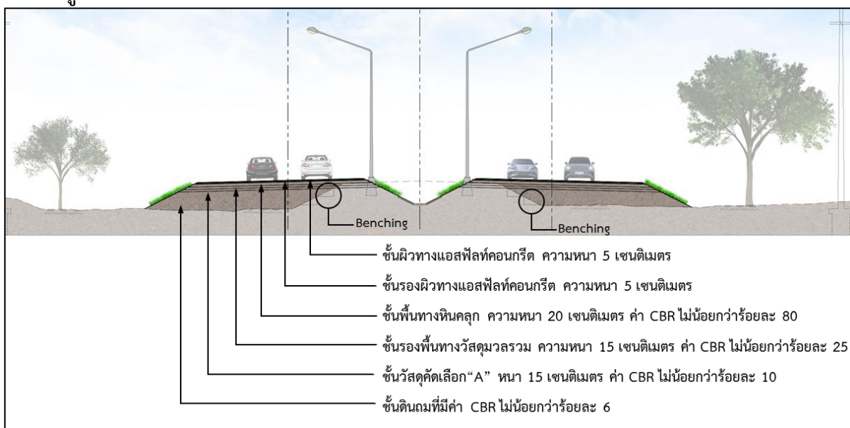
รูปที่ 5.1-4 รูปแบบโครงสร้างชั้นทาง
