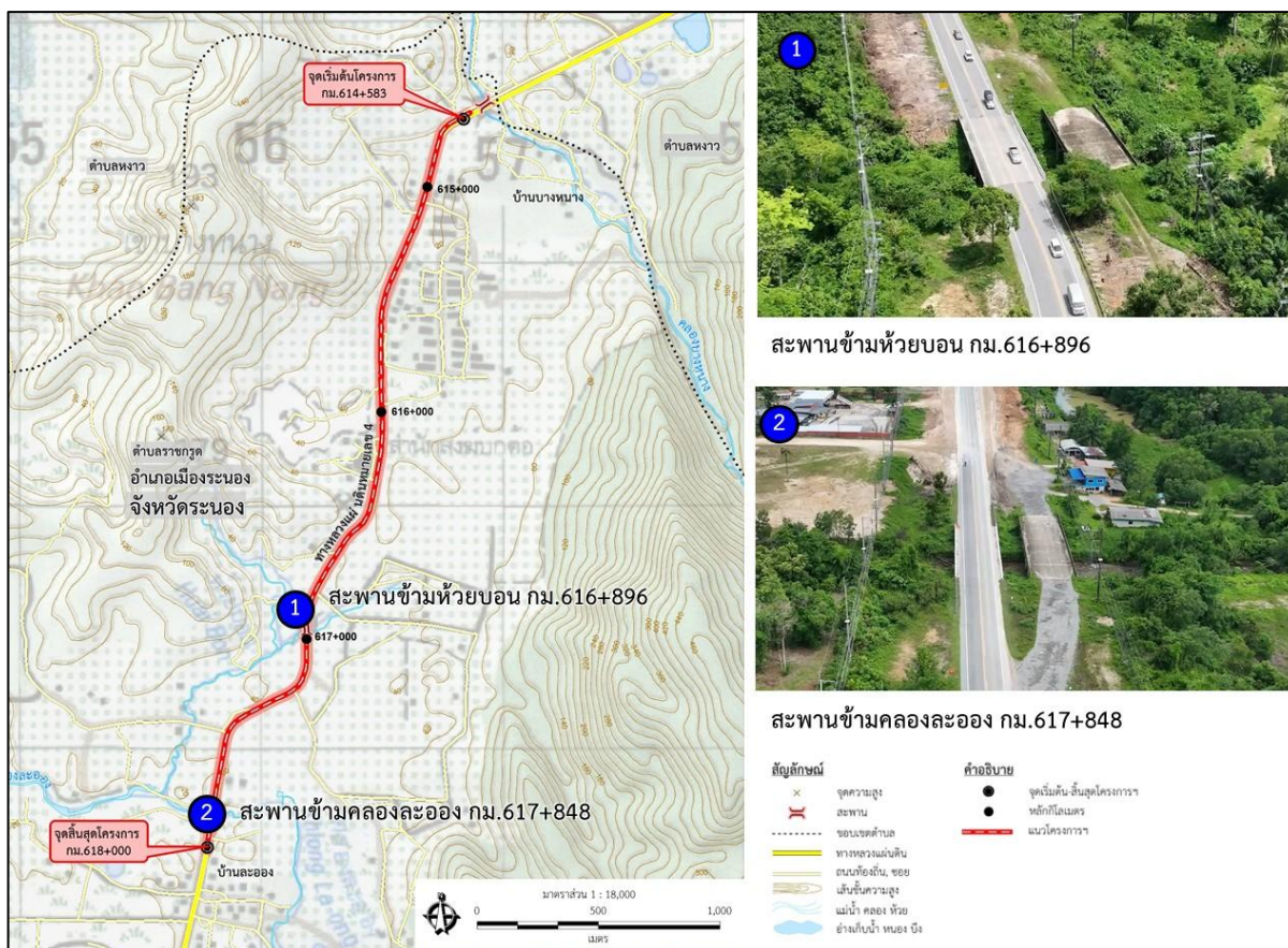
รูปที่ 5.1-8 ตำแหน่งและสภาพสะพานโครงการปัจจุบัน
