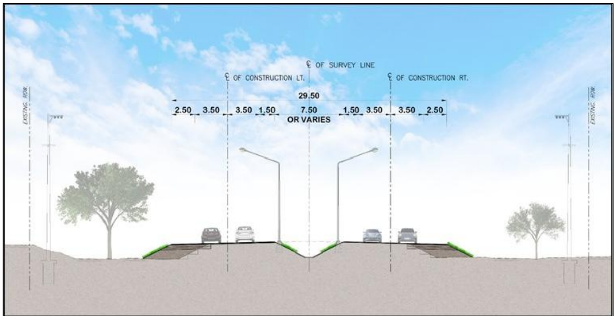
รูปที่ 5.1-2 รูปแบบก่อสร้างคันทางใหม่ทั้งสองข้าง
