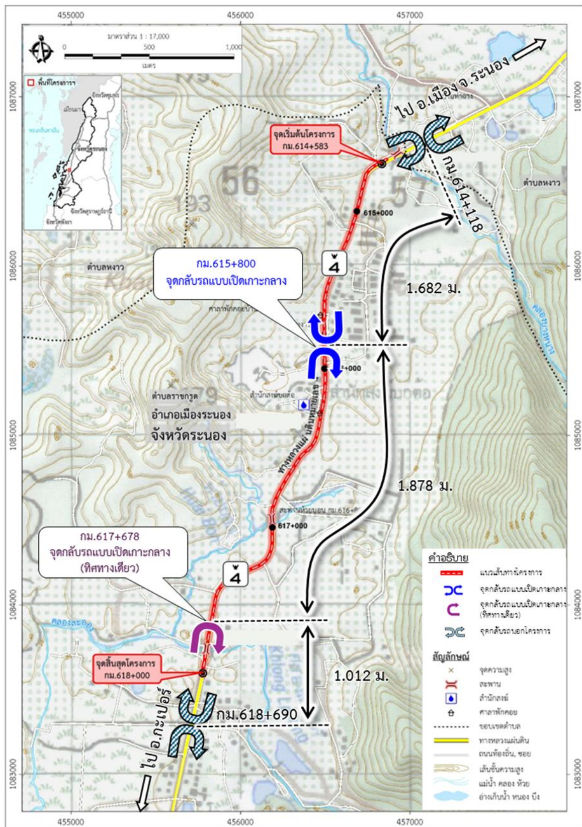
รูปที่ 5.1-6 ตำแหน่งจุดกึ่งกลางโครงการ
