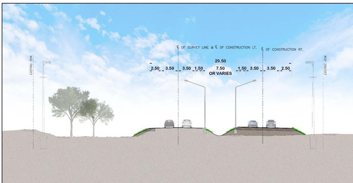
รูปที่ 5.1-3 รูปแบบก่อสร้างคันทางใหม่ ด้านขวาทางของคันทางเดิม
